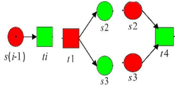
b) Redes de Petri
